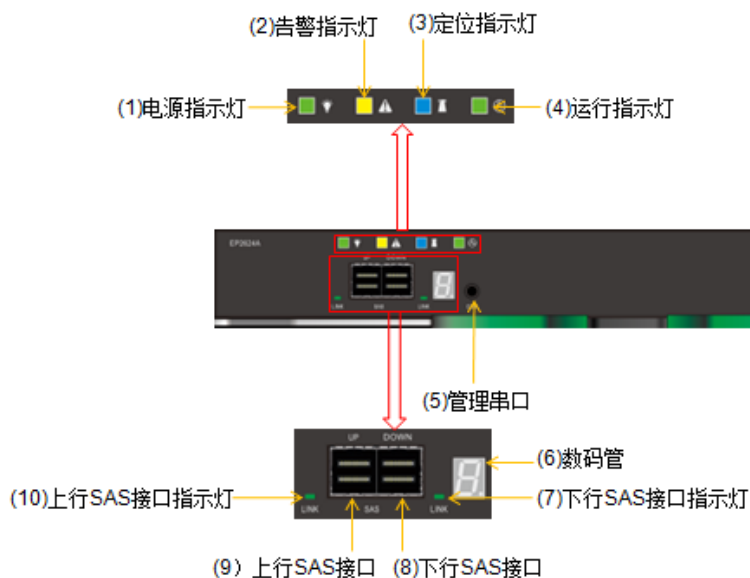
图3-14 DSU2624 的 EP 正视图
