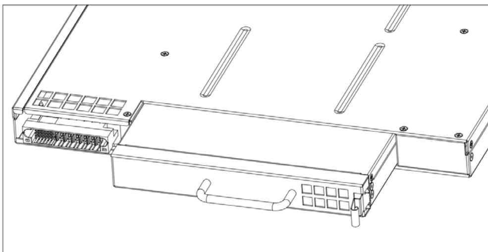
图6-6 安装/拆卸电池模块示意图
