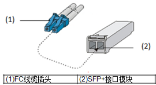
图4-33 FC 线缆和接口示意图
