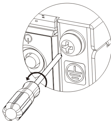
图4-21 松开设备接地端子的螺钉示意图
