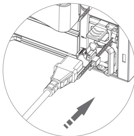
图4-24 安装电源线示意图（二）
