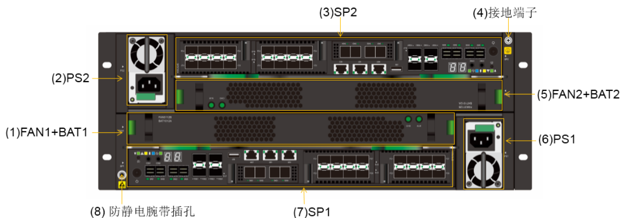
图3-2 SPU 后正视图
