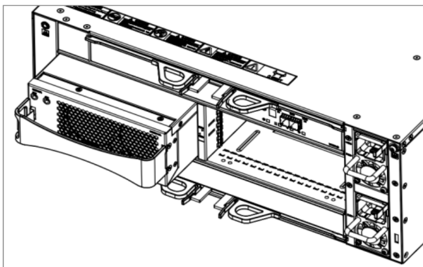
图6-8 安装/拆卸 DSU2624 风扇模块示意图
