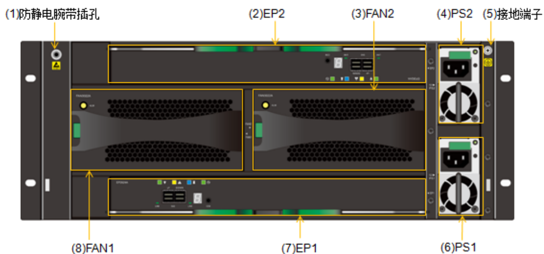
图3-13 DSU2624 后正视图
