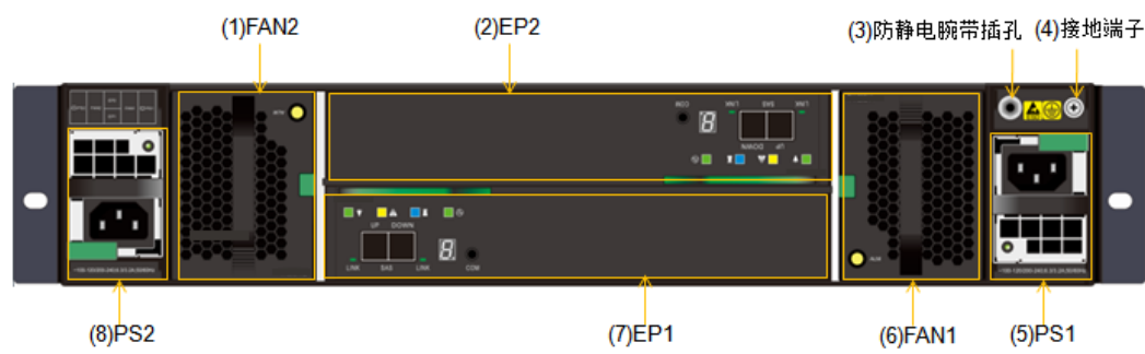
图3-8 DSU2625 后正视图
