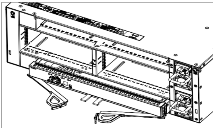
图6-3 安装/拆卸 DSU2624 EP 示意图
