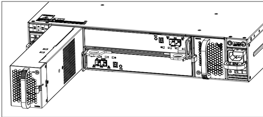
图6-7 安装/拆卸 DSU2625 风扇模块示意图
