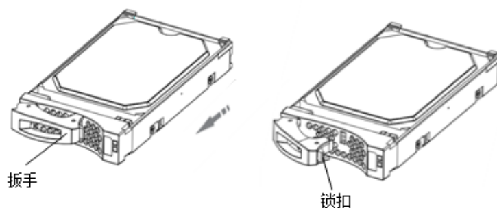
图6-18 安装 3.5 英寸磁盘模块示意图（一）
