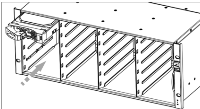
图6-19 安装 3.5 英寸磁盘模块示意图（二）
