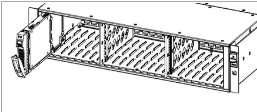
图6-15 安装 2.5 英寸磁盘模块示意图（二）
