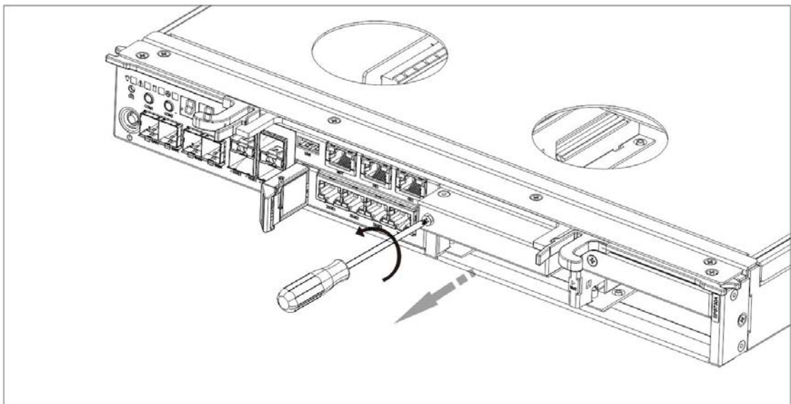
图6-11 拆卸挡板示意图
