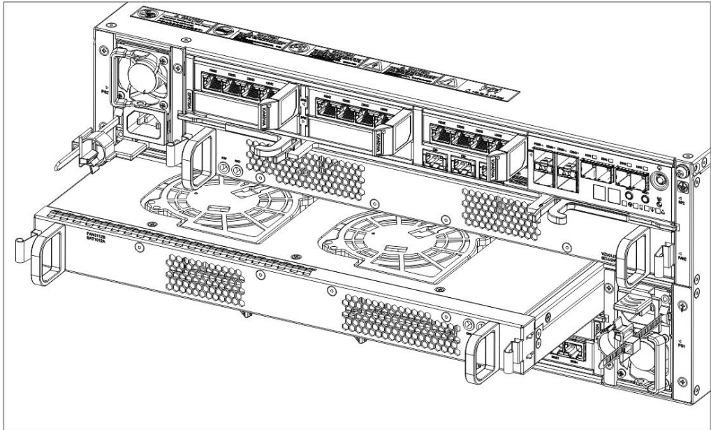
图6-5 安装/拆卸 SPU 风扇模块+电池模块示意图
