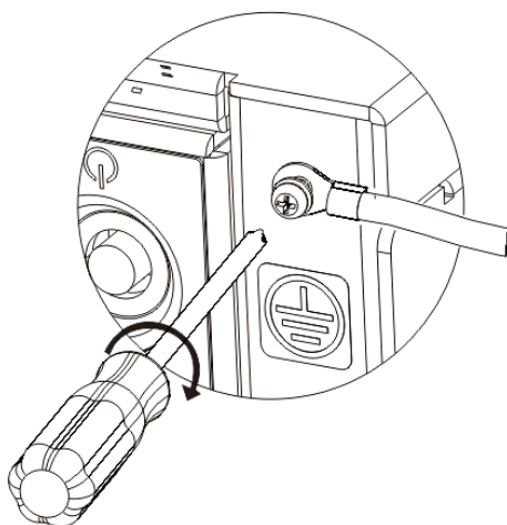
图4-22 安装接地线示意图
