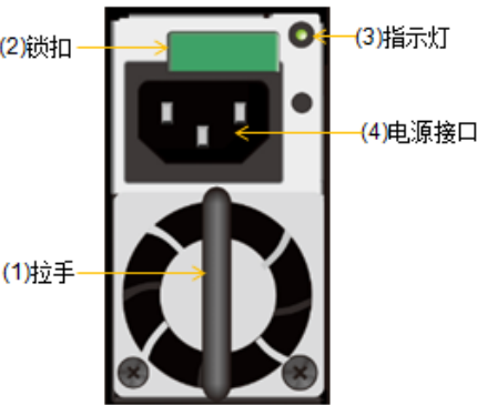
图3-16 DSU2624 电源模块正视图
