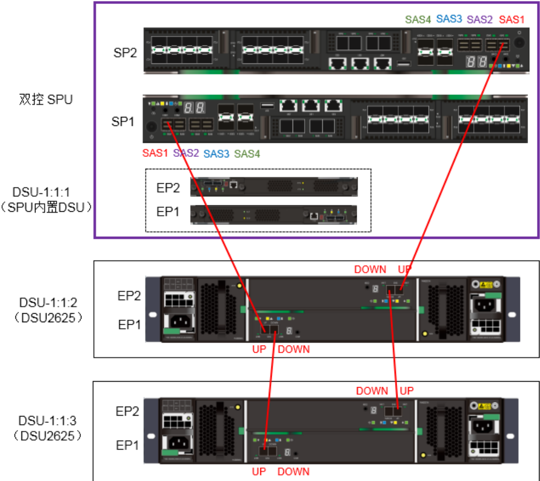
图4-31 SAS 线缆安装示意图
