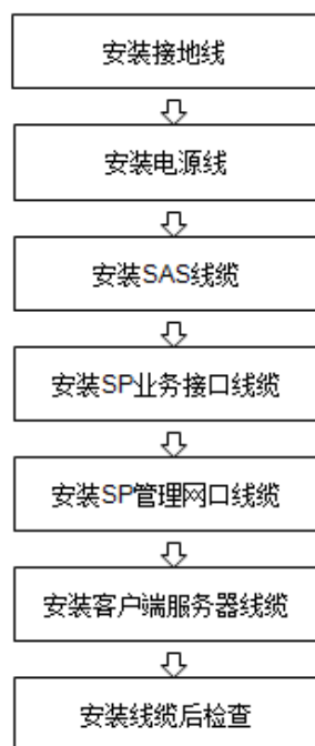
图4-19 线缆安装流程示意图
