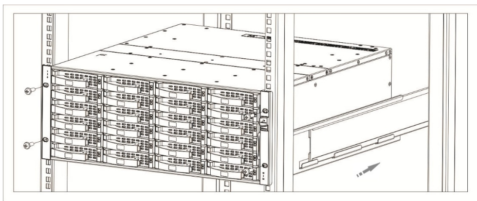
图4-12 安装 SPU 示意图
