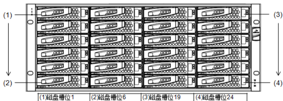
图6-17 SPU/DSU2624 磁盘槽位编号示意图
