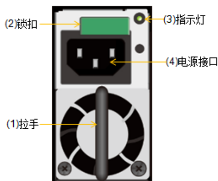
图3-6 SPU 电源模块正视图
