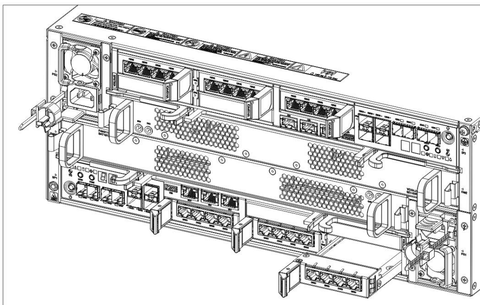
图6-9 安装/拆卸 IO 插卡小卡示意图
