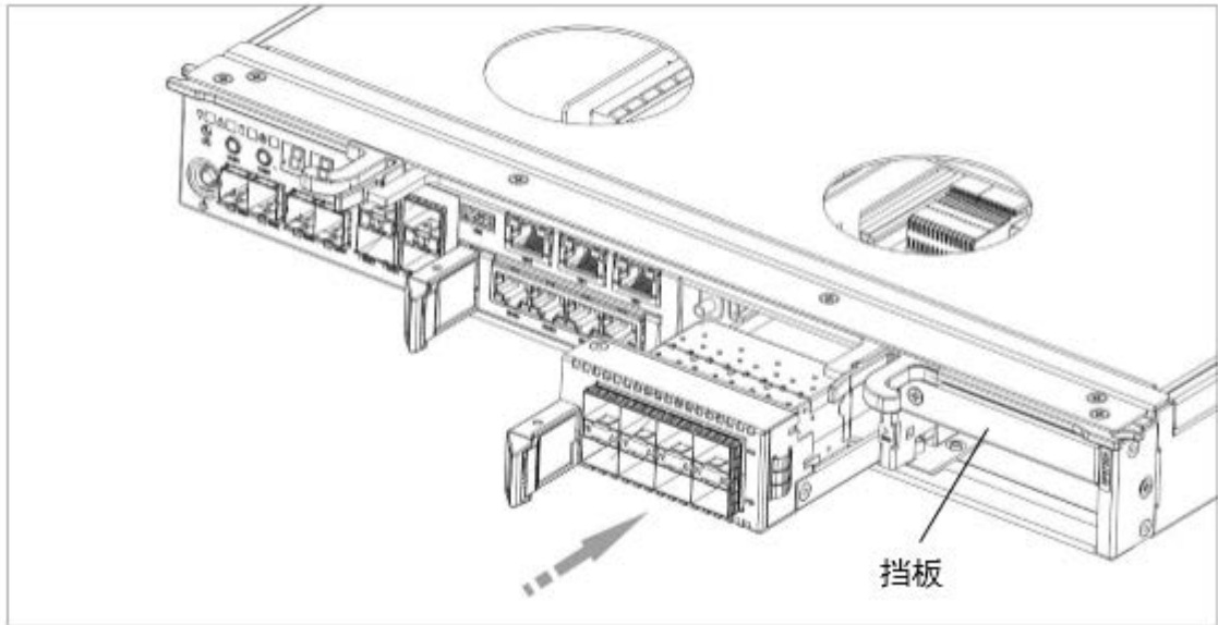
图6-10 安装/拆卸 IO 插卡大卡示意图
