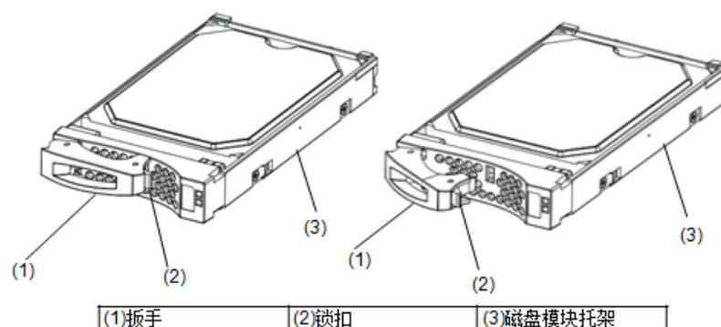
图6-16 3.5 英寸磁盘模块示意图
