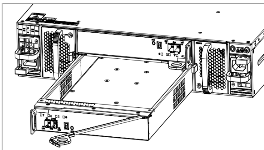
图6-2 安装/拆卸 DSU2625 EP 示意图
