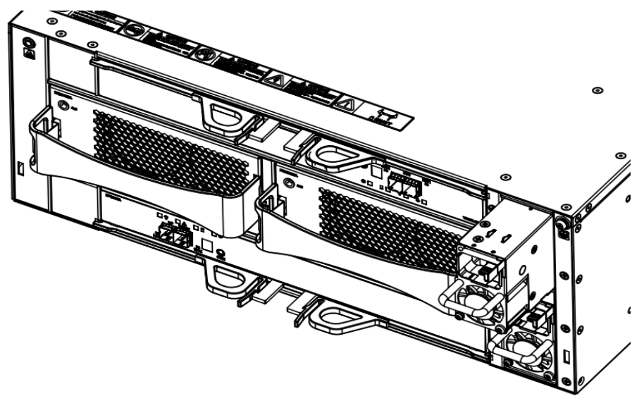
图6-4 安装/拆卸 DSU2624 电源模块示意图
