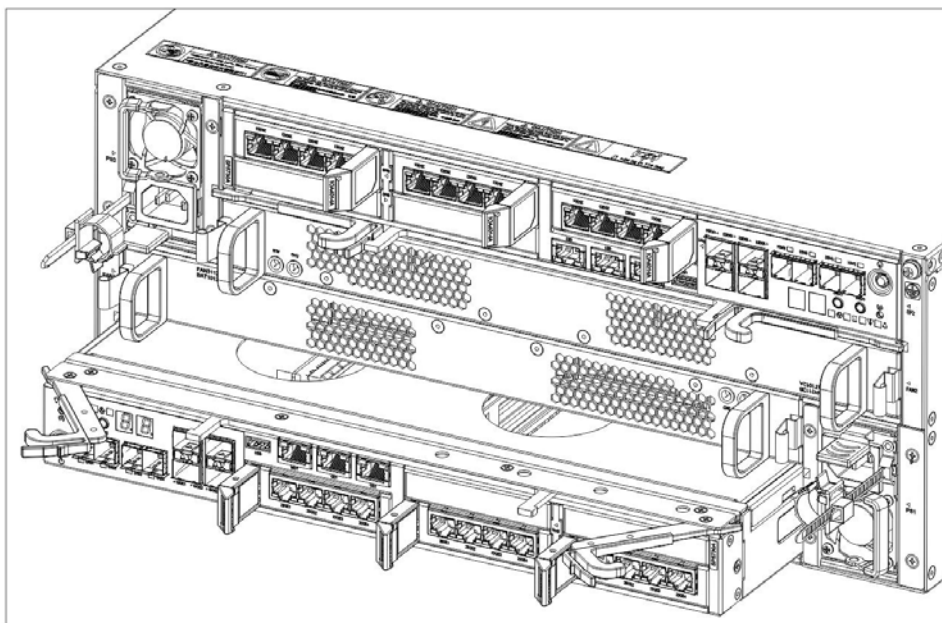
图6-1 安装/拆卸 SP 示意图
