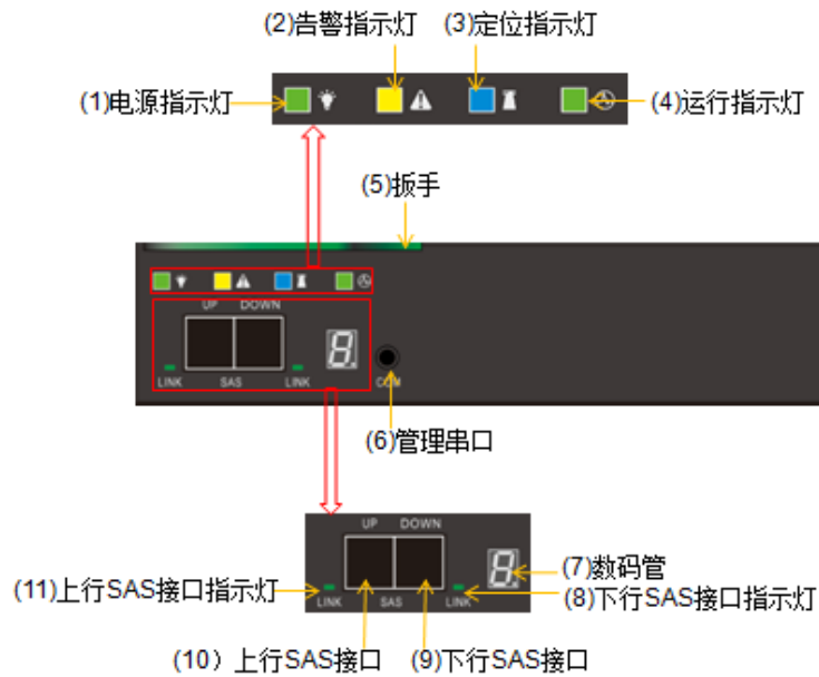
图3-9 DSU2625 的 EP 正视图
